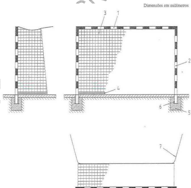
Figura 1 e 2: Exemplo Baliza de Andebol do tipo 1
