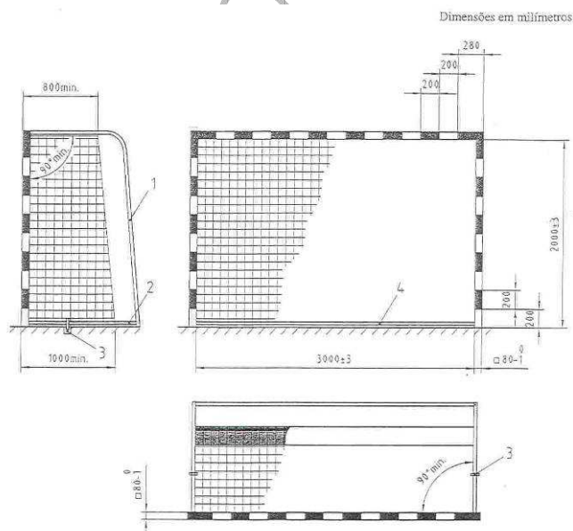
Figura 3 e 4: Exemplo Baliza de Andebol do tipo 2
